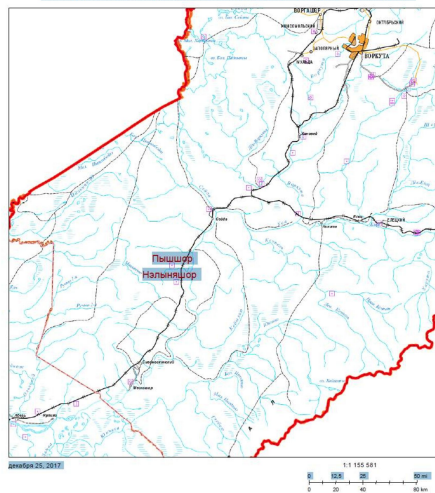
Схема расположения месторождений Пышшор, Нэлыняшор
